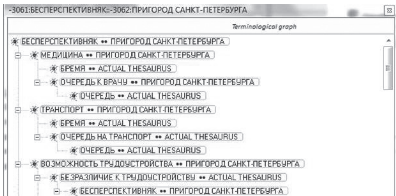
Рис. 5. Терминологический граф
